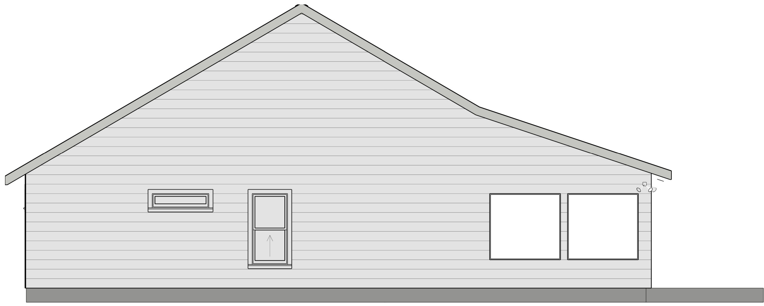
Right Elevation
